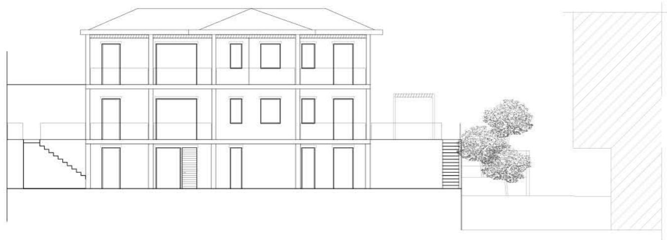
Recupero residenziale dell'edificio in Via Dondo degli Infanti, 6 - Varazze
